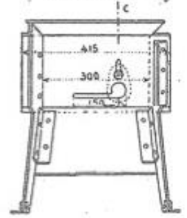
Fig. 95. — Abri blindé pour guetteur, type S. T. G.
