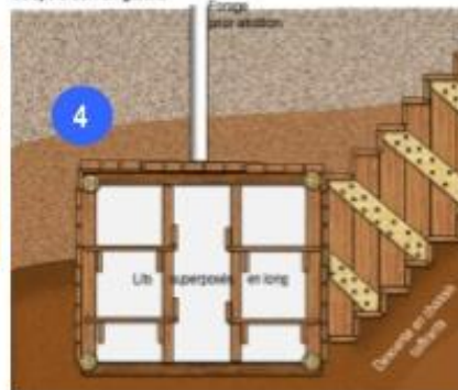
Coupe d'abri en galerie
