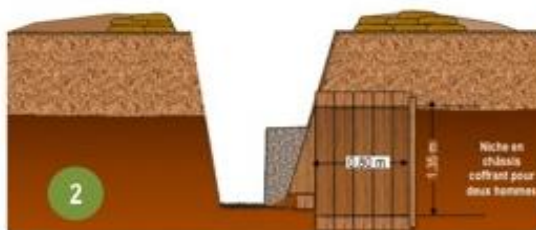
Abri de paroi
